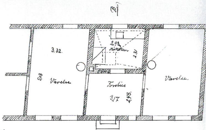
Grundplan
