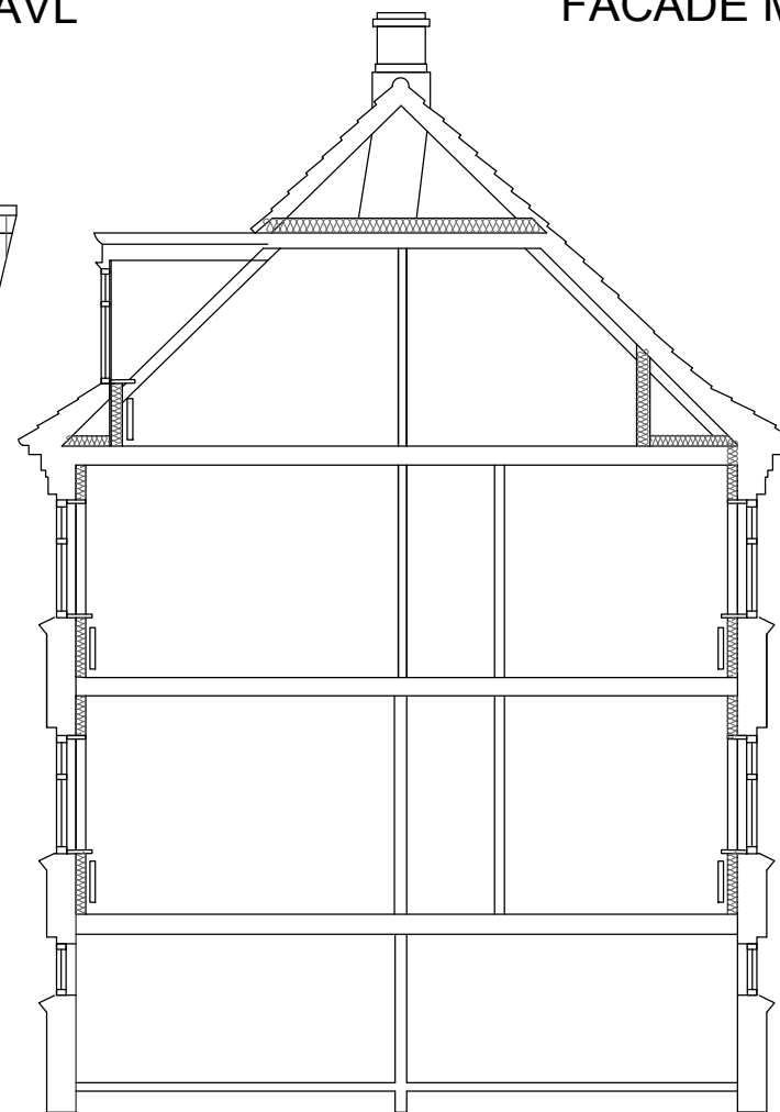
SNIT A-A
