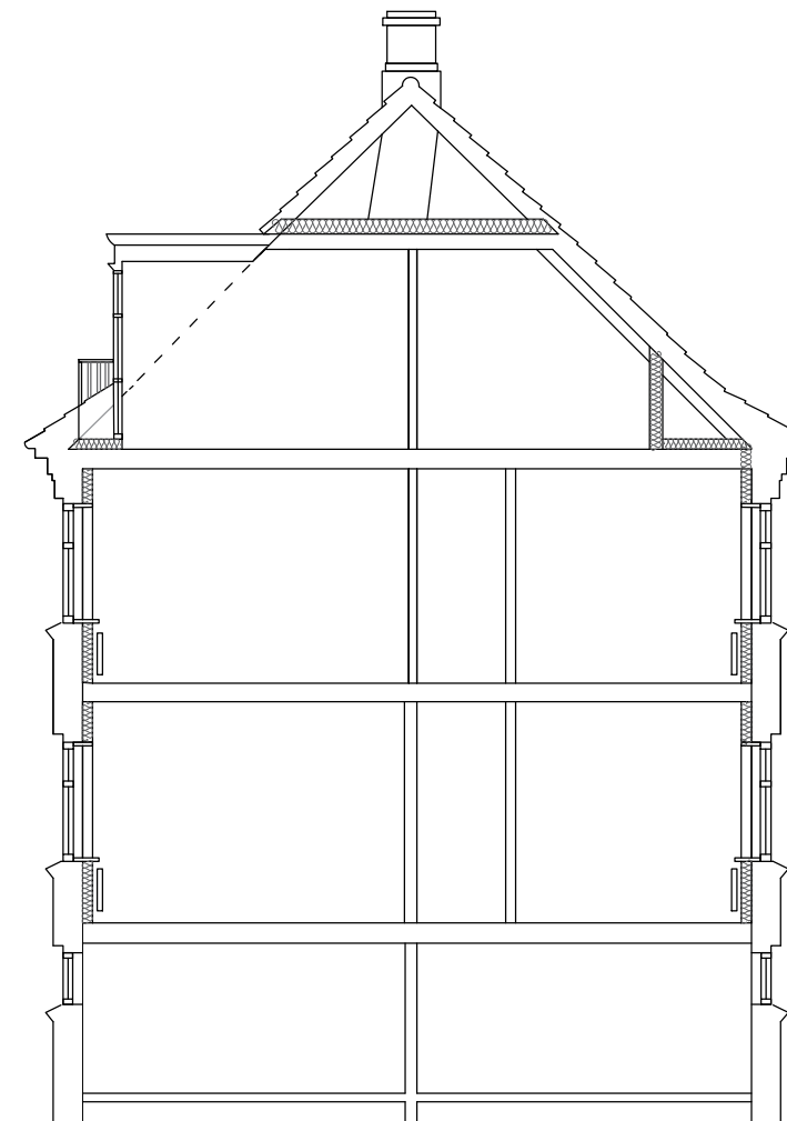
SNIT A-A
