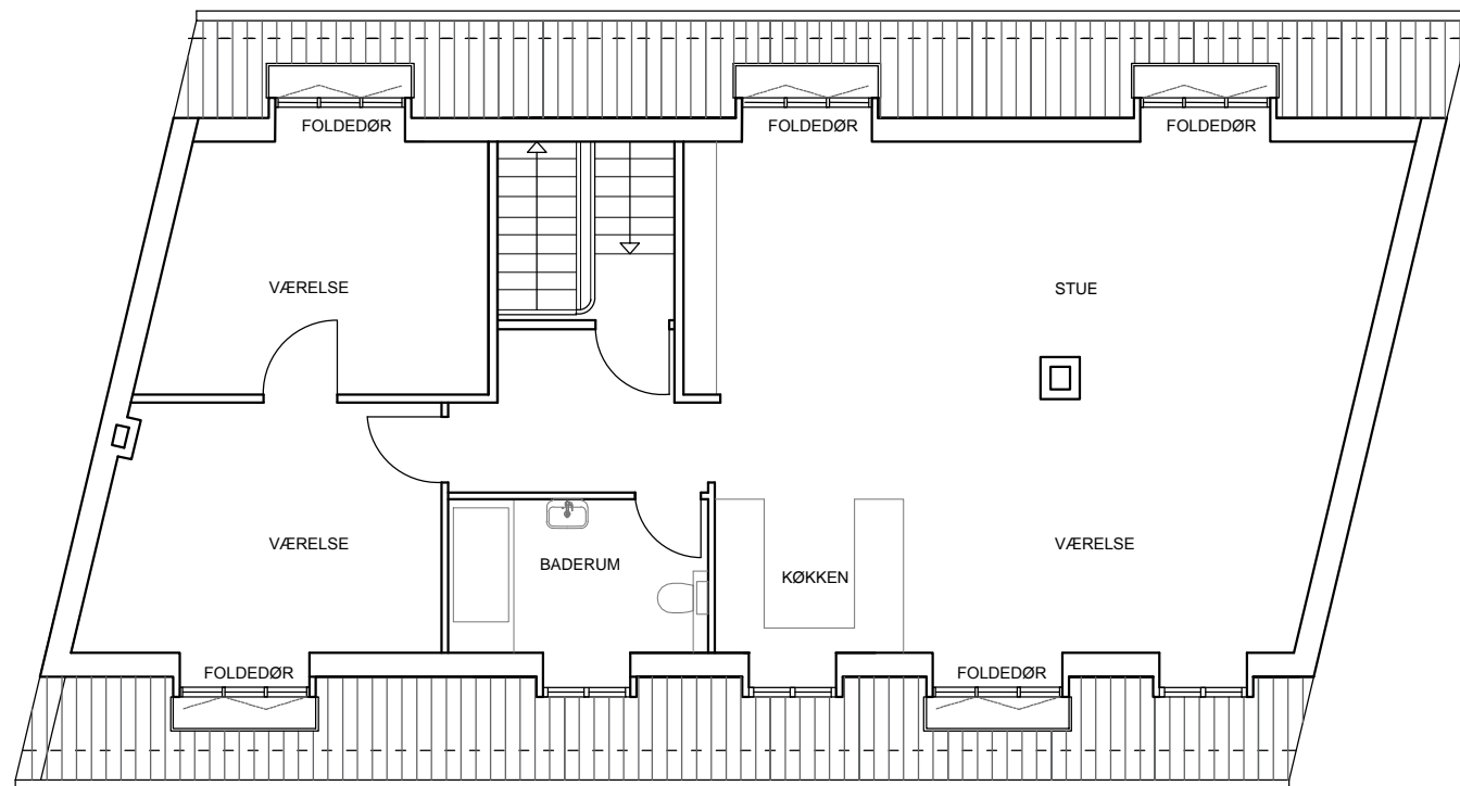
TAGETAGE PLAN
