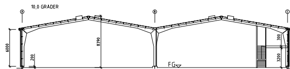
SEKTION A-A
