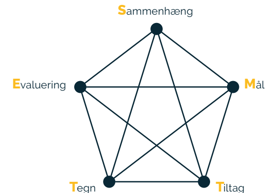
Figur 1: SMTTE-model
