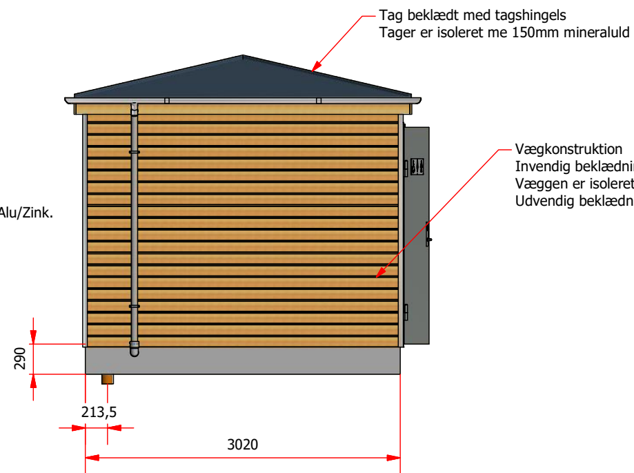
A-A ( 1 : 10 )
