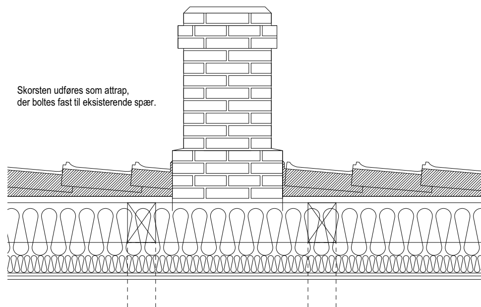
Længdesnit i tag med opstalt af skorsten
