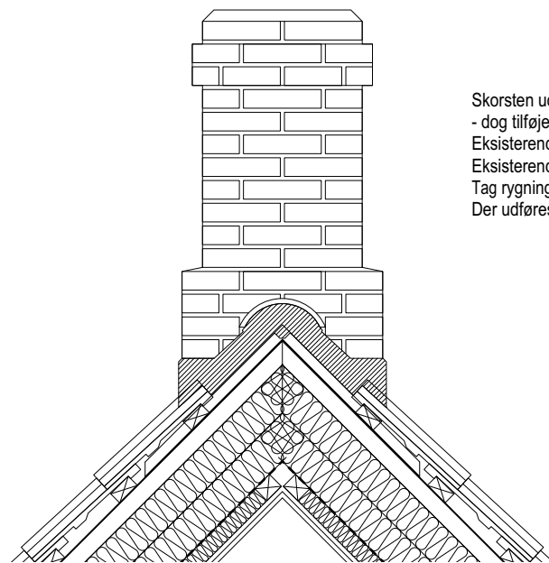
Tværsnit i tag med inddækninger i mørtel
