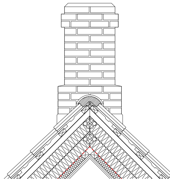
Tværsnit i tagrygning med opstalt af skorsten
