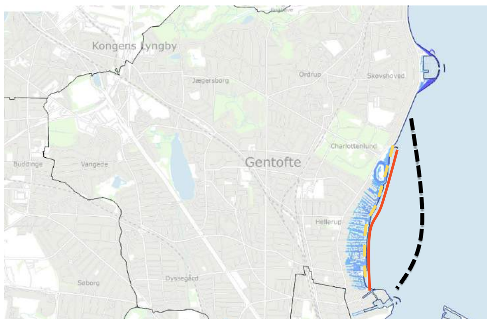
Figur 9-1 Illustration af de arealer der er mest udsat for oversvømmelser og skitsering af mulige sikringstyper for Gentofte. Gul stilet: sikring af enkeltejendomme, rød: gennemgående sikring, sort: gennemgående sikring i vandet. (SCALGOlive).
